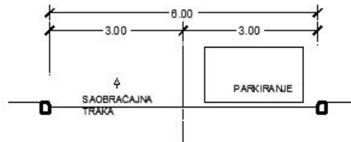
PROFIL JEDNOSMJERNE ULICE
