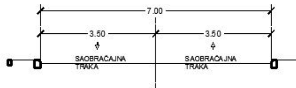
PROFIL DVOSMJERNE GRADSKE ULICE
