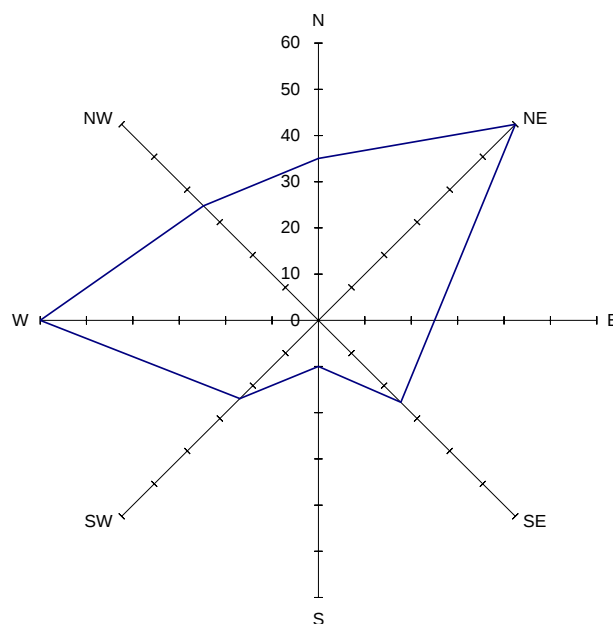
Ilustracija 2 - Ruža vjetrova za grad Srebrenik
