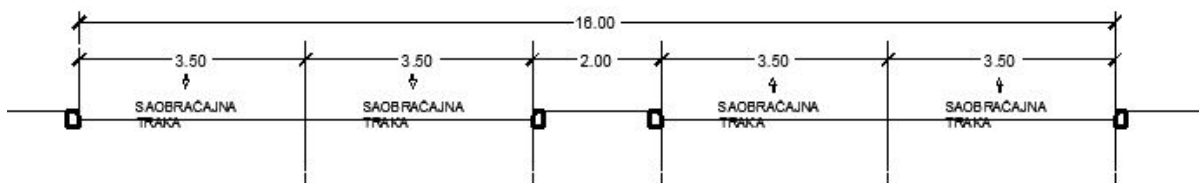
PROFIL REGINALNE CESTE
