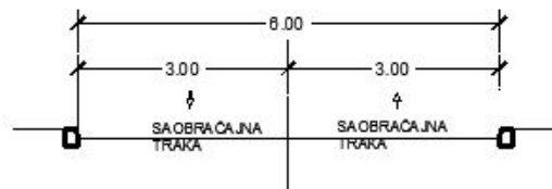
PROFIL JEDNOSMJERNE ULICE SA PREDVIĐENIM PARKIRANJEM U JEDNOJ TRACI
