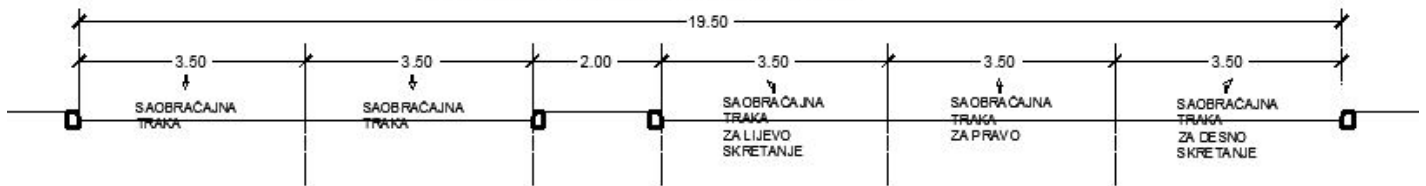
PROFIL GRADSKE SAOBRAĆAJNICE
